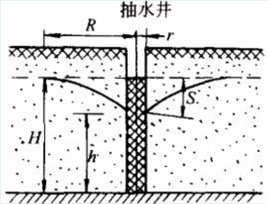
图 5.2.4 抽水试验井井孔示意图
