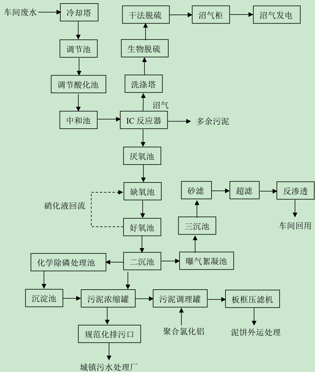
图 7.2.1 厂内污水处理站废水处理工艺流程图
