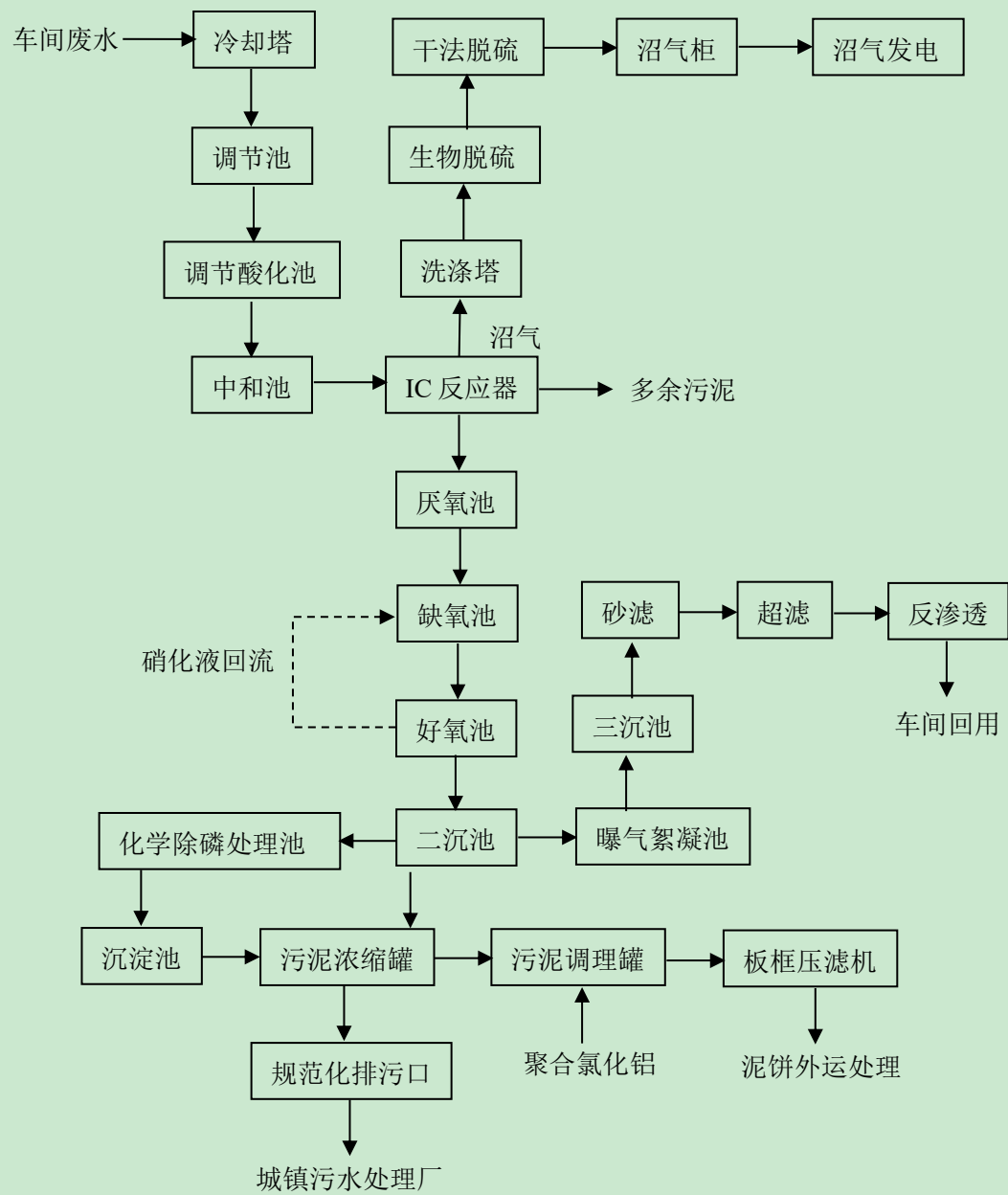
图 3.2.11 厂内污水处理站废水处理工艺流程图
