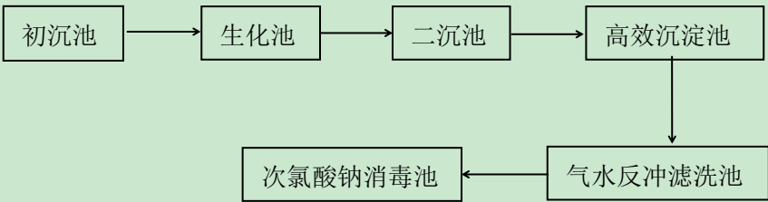
图 3.2.14 诸城市鑫兴污水处理厂二期工程处理工艺
