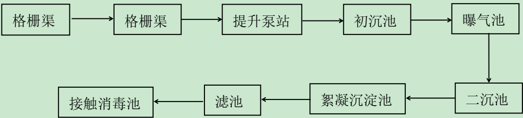
图 3.2.13 诸城市鑫兴污水处理厂一期工程处理工艺
