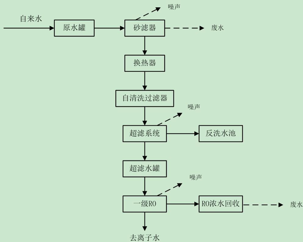
图3.2.6 纯水制备工艺流程图
