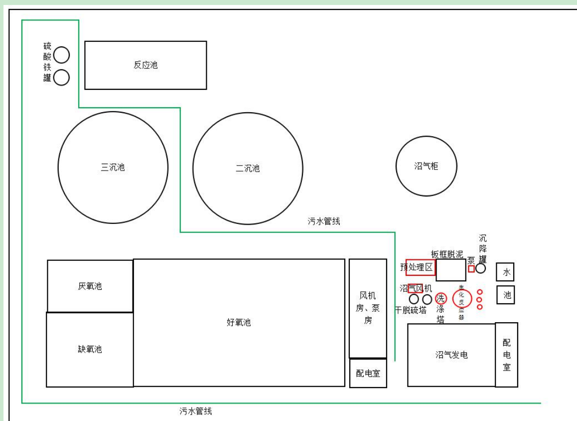
图 3.2.12 厂内污水处理站平面布置示意图
