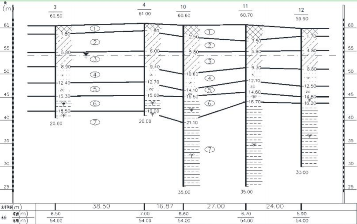
图 5.2.3 项目建设区工程地质剖面图
